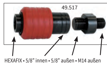
49.517 HEXAFIX • 5/8" innen • 5/8" außen • M14 außen
